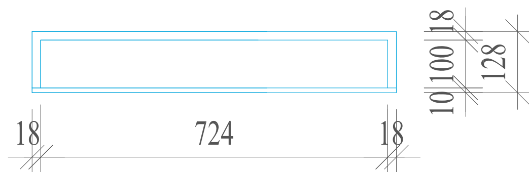
Вид сверху
