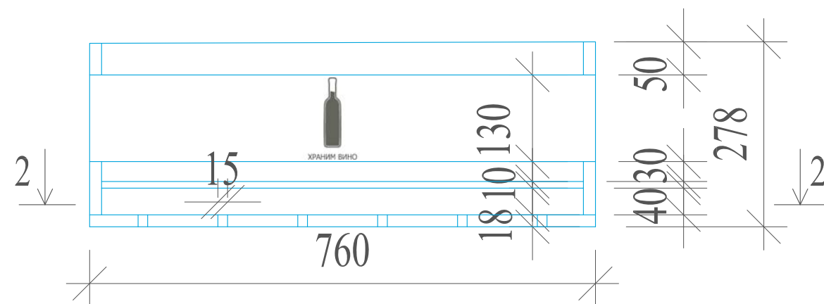
Вид спереди
